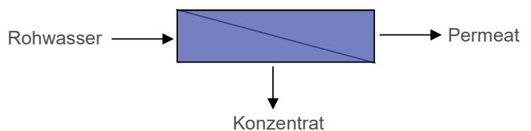
Membranmodul, Schema
